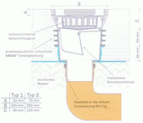
KRASO® Hofablauf Typ 1
