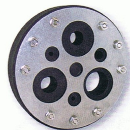
4 KRASO® Typ 200 M Ausführung: 1 Beispiel: 1 x 38 mm 1 x 26 mm 1 x 22 mm 1 x 12 mm 2 x 6 mm 1 x Blind
