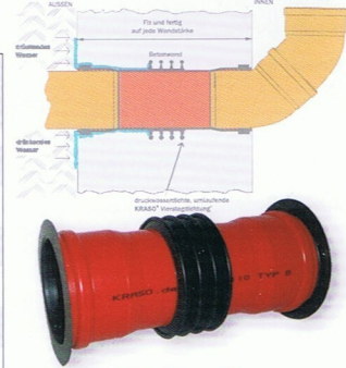
KRASO® Typ B
