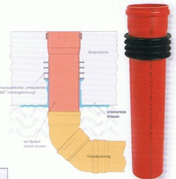
KRASO® Typ BDF
