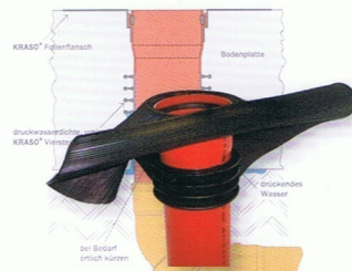
KRASO® Typ BDF mit Folienflansch
